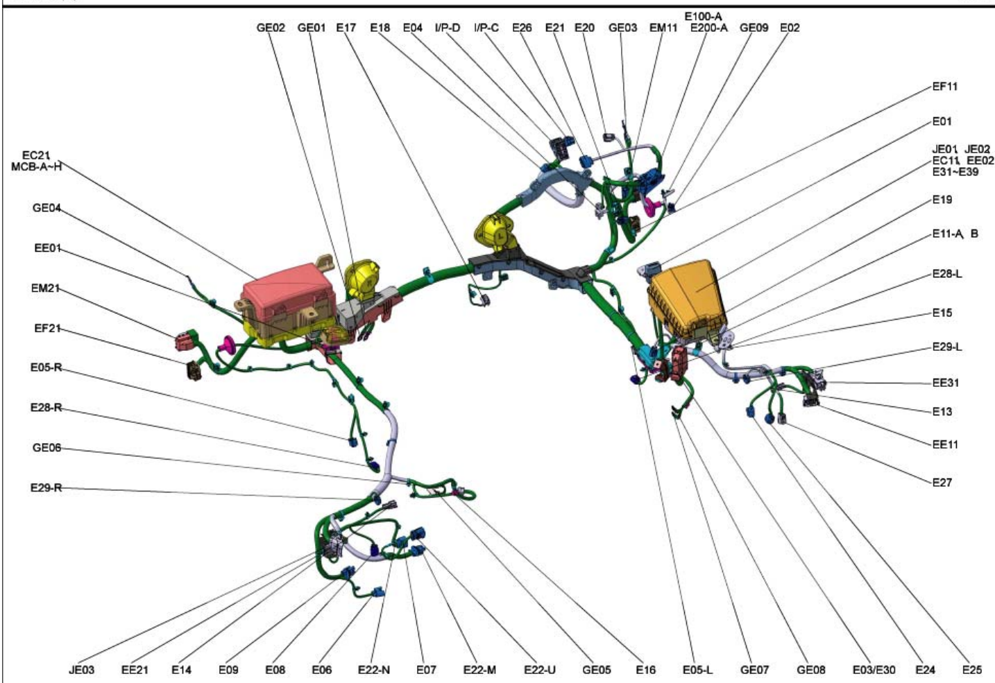
前线束(1)
